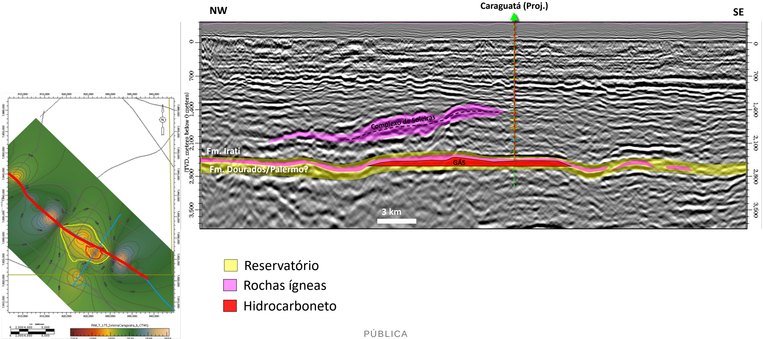
Seção sísmica em Profundidade com interpretação - Inline
