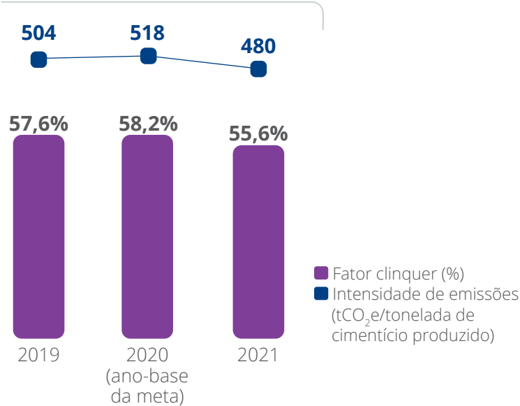
Intensidade de emissões do segmento Cimentos (kgCO 2 e/tonelada de cimentício)
