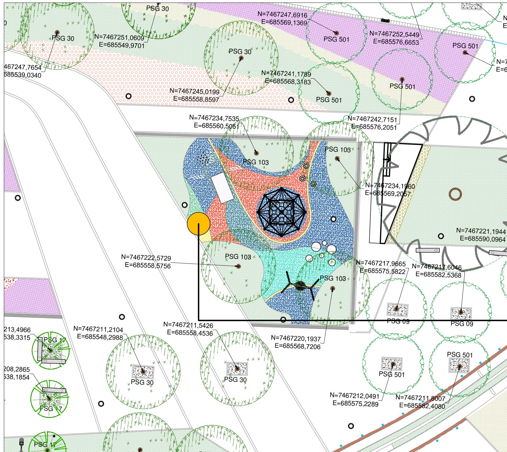
PLANTA DE SITUAÇÃO PRAÇA MUHAMMAD ALI - ESCALA 1/150
