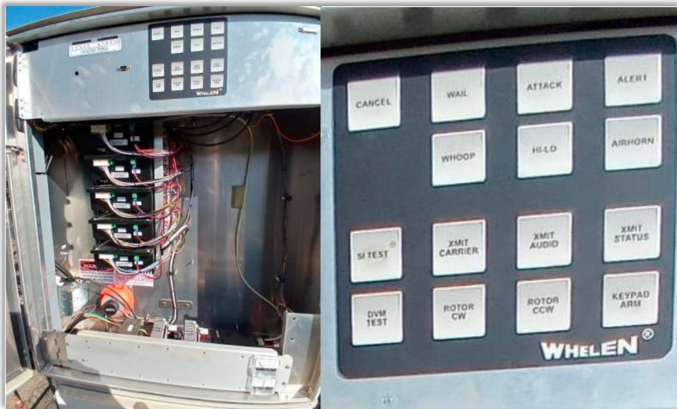
Figura 7: Painel de acionamento torre Whelen_Fig1 Teclado local torre Whelen
