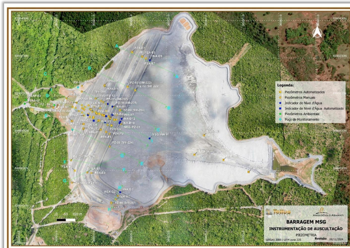
Figura 37: Localização dos piezômetros e indicadores de nível d'água na estrutura
