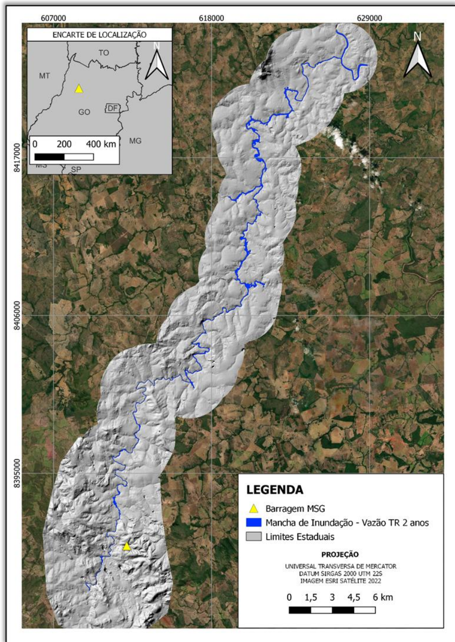
Figura 19: Envoltória da modelagem de vazão natural para TR de 2 anos no MDT tratado.
