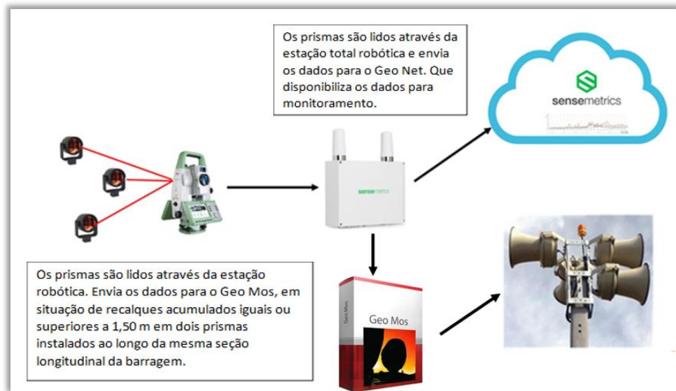
Figura 3: Esquemática de acionamento automático das sirenes
