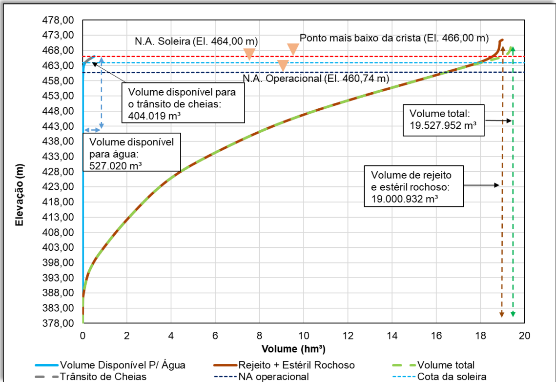
Figura 15: Curva cota-volume da Barragem MSG
