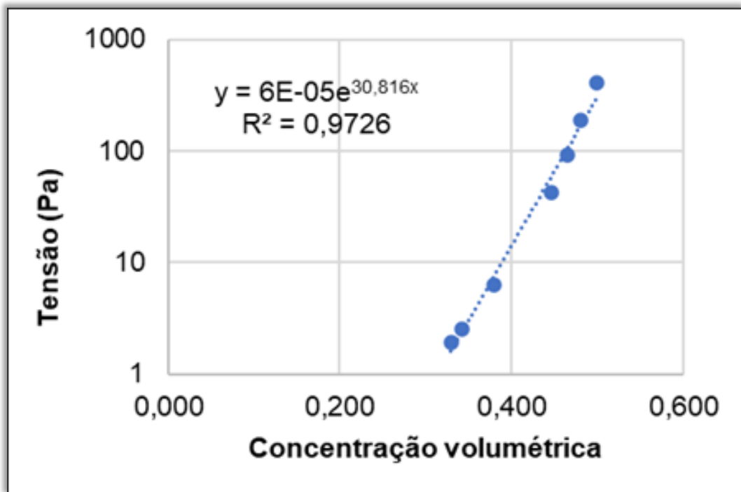
Figura 16: Tensão limite de escoamento em função da concentração volumétrica da mistura – Amostra AdoB585
