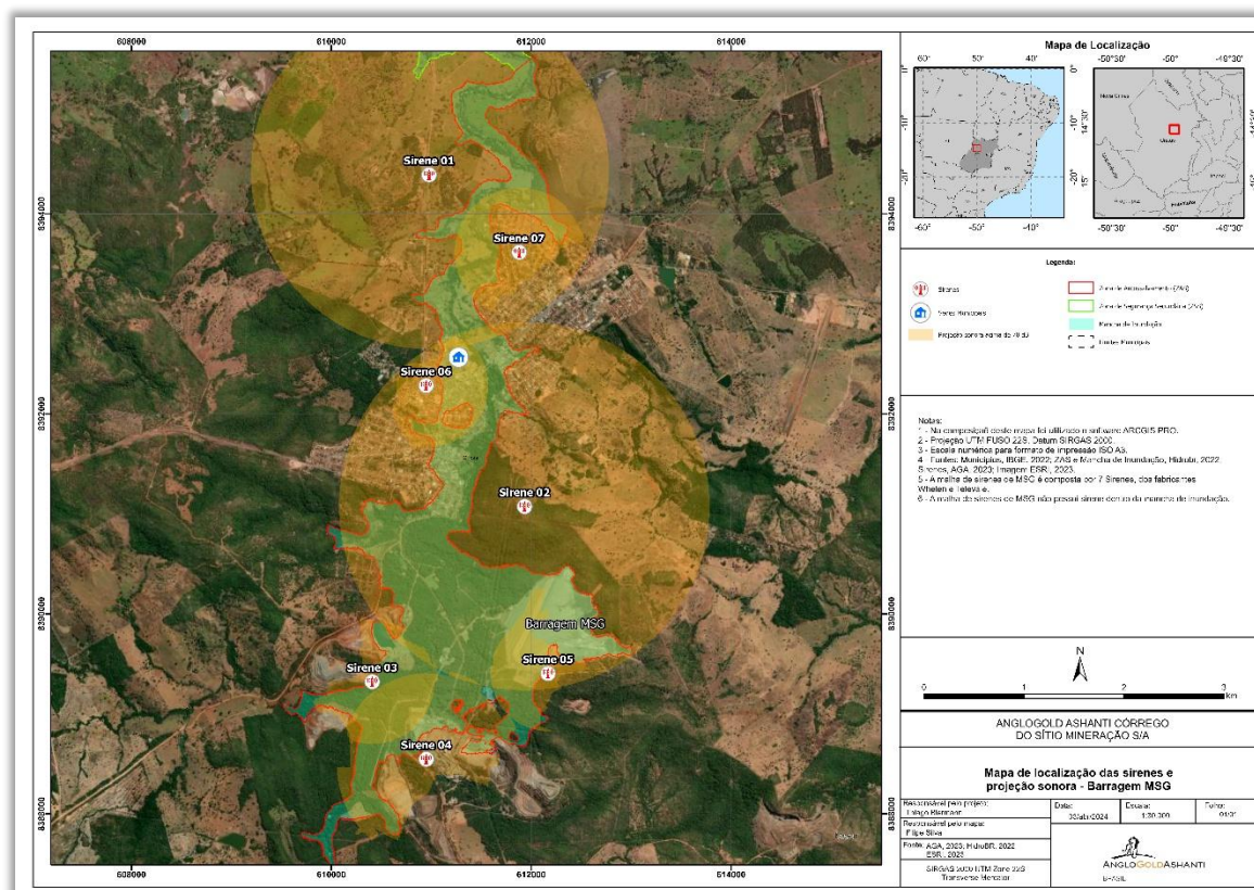
Figura 12: Posição das sirenes no campo
