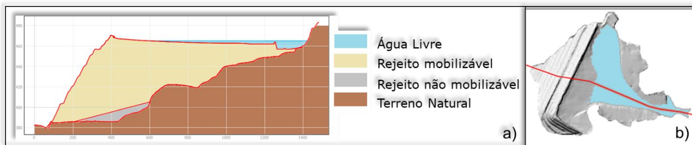
Figura 18: Representação gráfica do volume mobilizável – Ruptura Extrema
