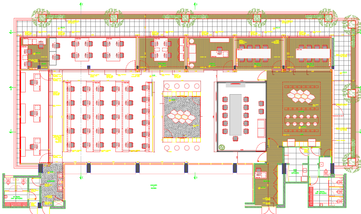
PLANTA LAYOUT esc.: 1/50
