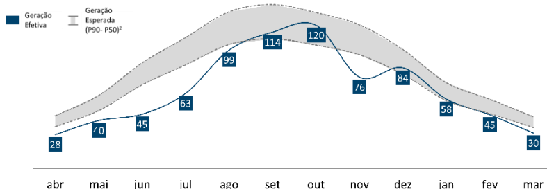
Geração (MWm)
