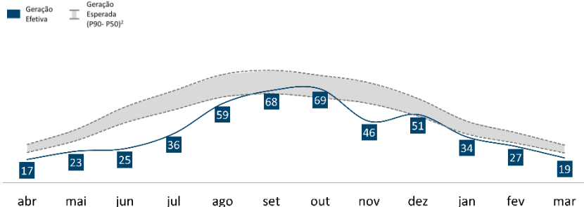
Geração (MWm)
