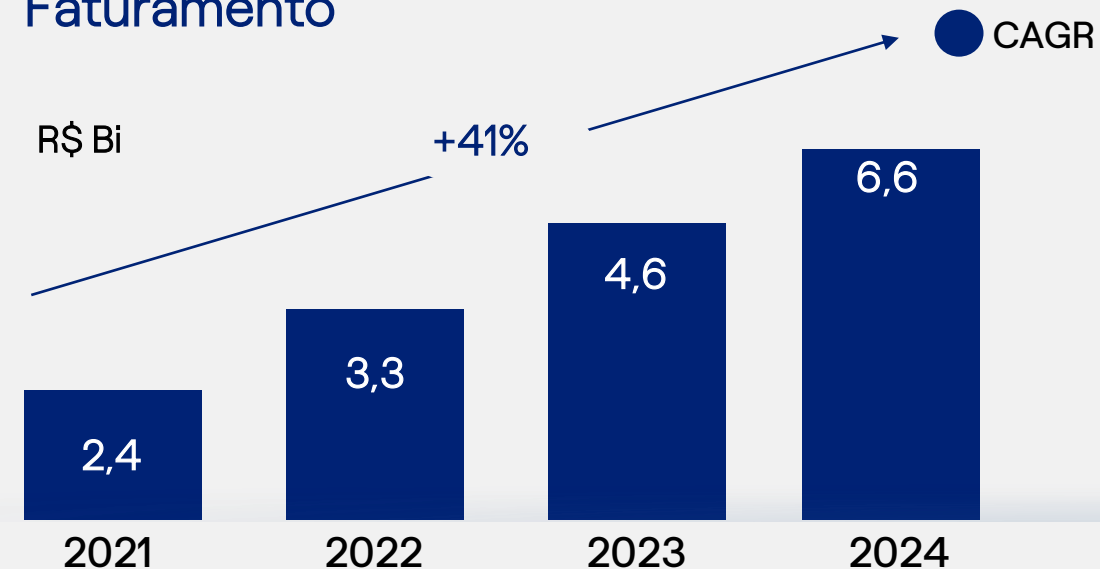
Faturamento
