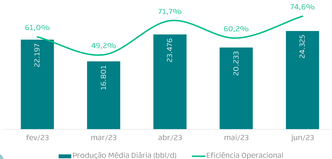
Produção Média Diária (net PRIO) e Eficiência Operacional Albacora Leste
