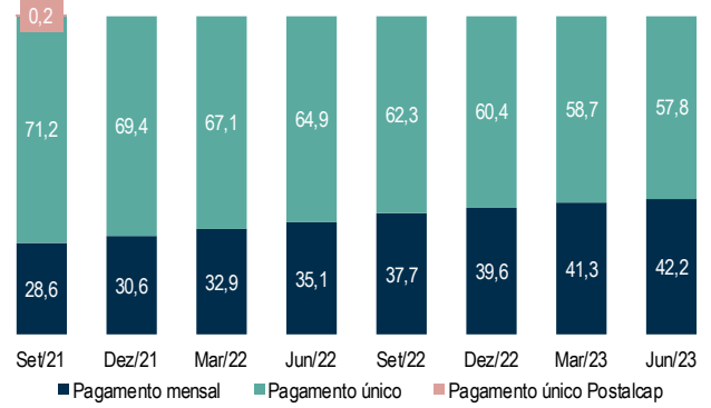
Figura 58 – Brasilcap | Títulos ativos por produto (%)
